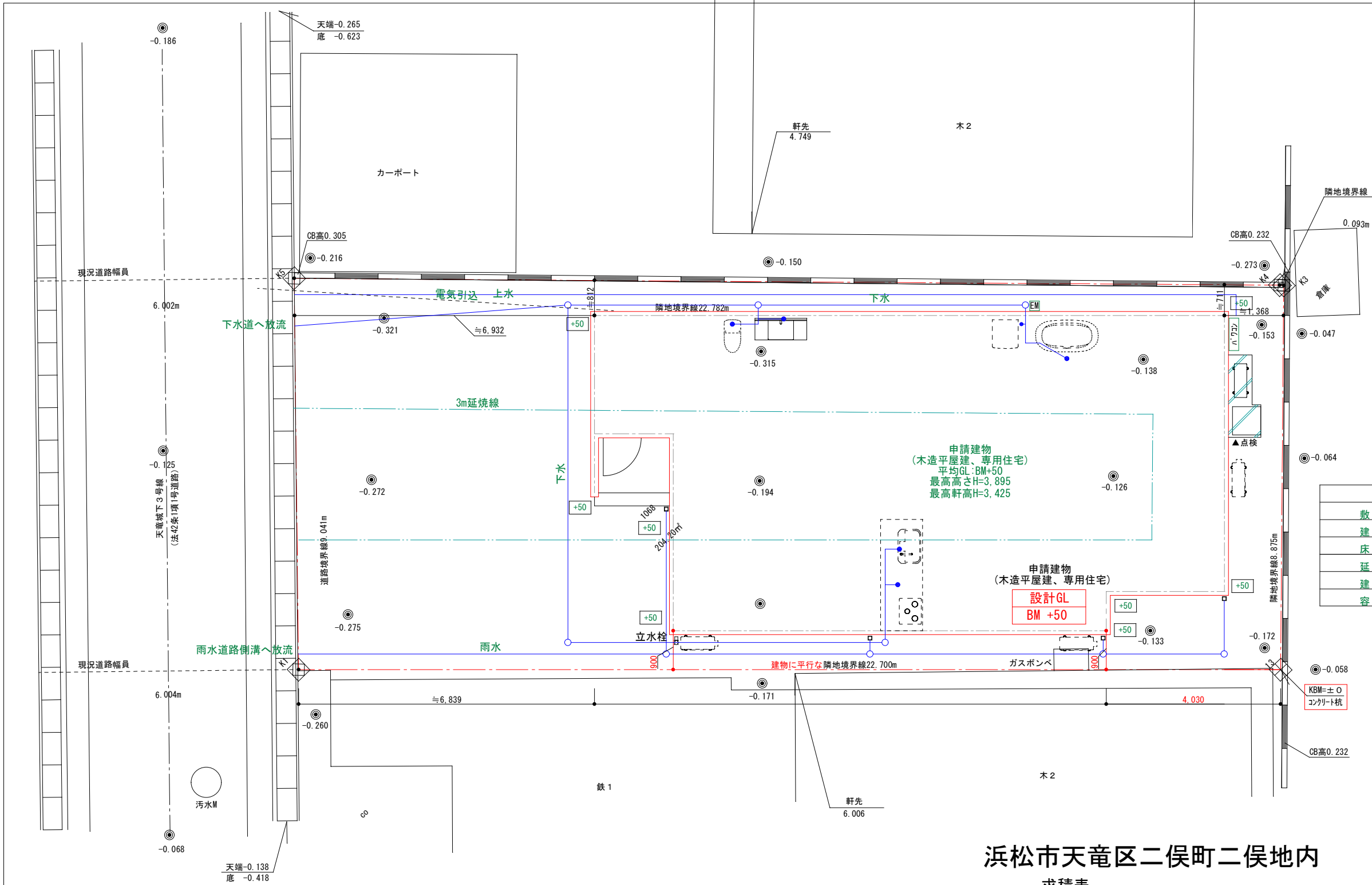
求積図 (1/250)
