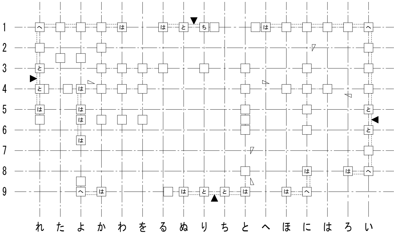
1 階柱壁伏図
