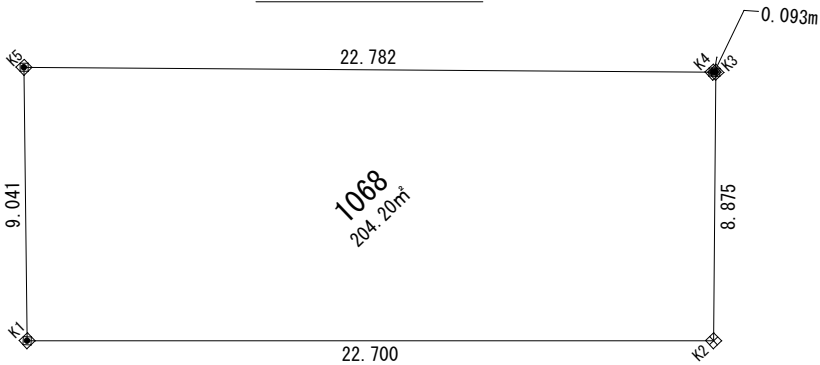
求積図 (1/250)
